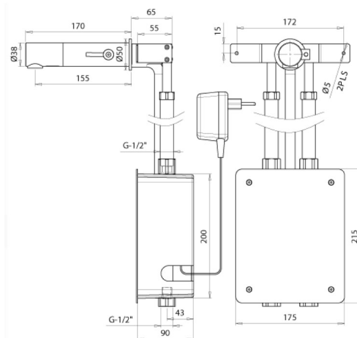
Versione a trasformatore (RUEL07ME).
